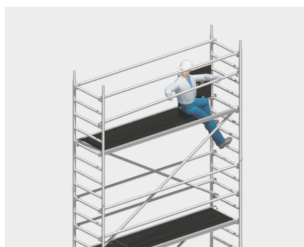
Nachrüstkit für den Sicherheitsaufbau P2 für die Uni-Familie ab Seite 67
