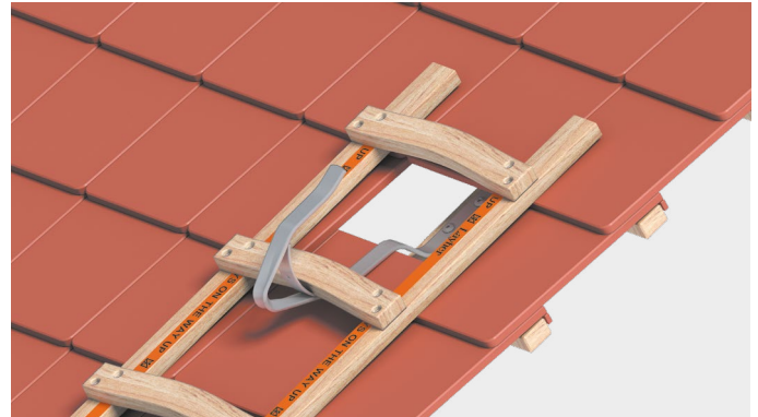
Beispielhafte Anwendung des Sicherheitsdachhakens Modell Z (Pos. 1)
