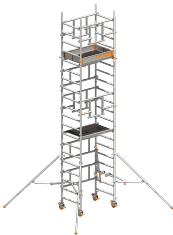
SoloTower P2 SAFETY PLUS mit Sicherheits-Doppelgeländer Seite 44
