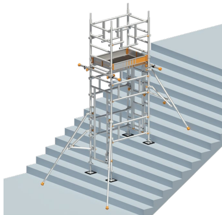
Treppen-Kit für den SoloTower P2 SAFETY PLUS mit Sicherheits-Doppelgeländer Seite 46
